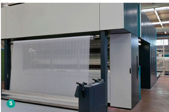
Back view of PROSIZE® Sizing Machine Rückansicht der PROSIZE® Schlichtemaschine
